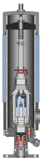
D-096-w (überflutbar!) BEV-Kompaktschacht mit D-46/2-Ventileinsatz
